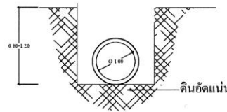
รูปตัดตามขวาง
