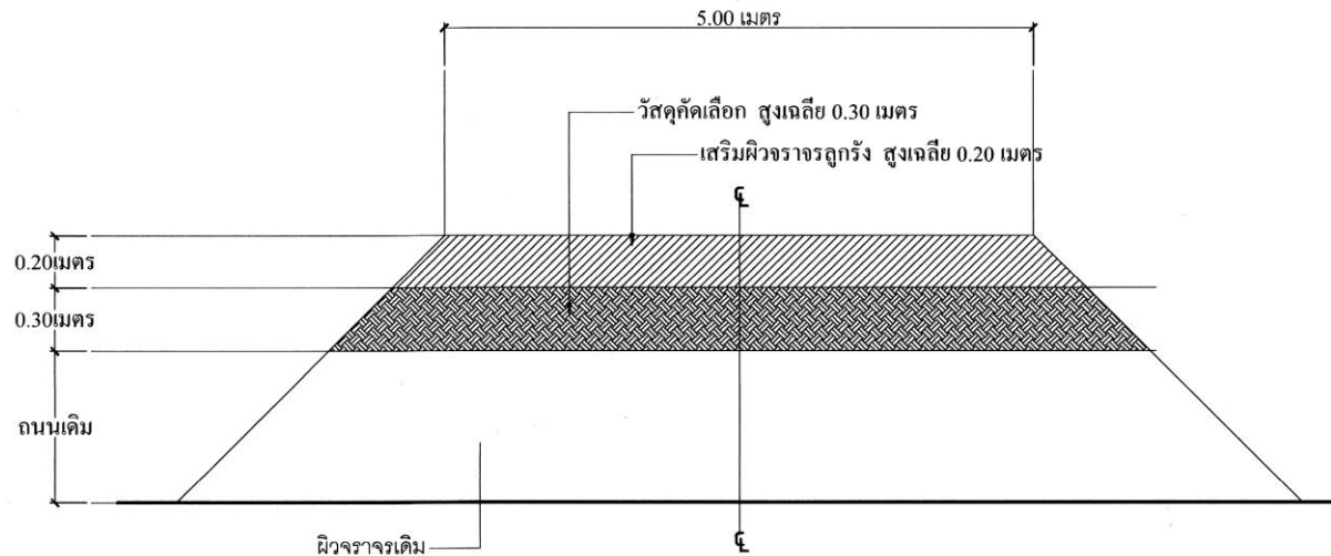
รูปตัด-ขยาย ถนนลูกรัง (ช่วงที่ 1)
