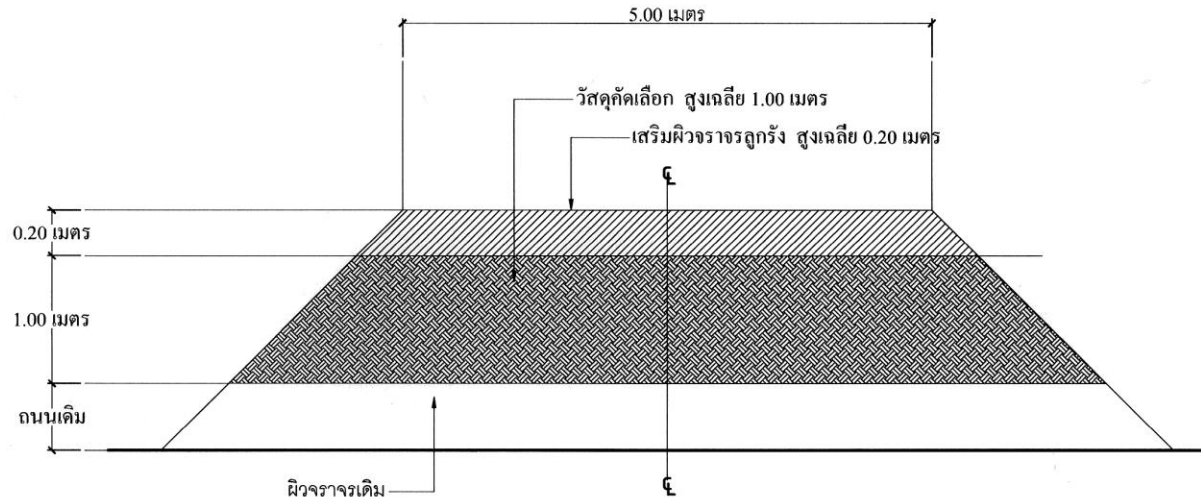
รูปตัด-ขยาย ถนนลูกรัง (ช่วงที่ 2) 0+350 ถึง 0+830
